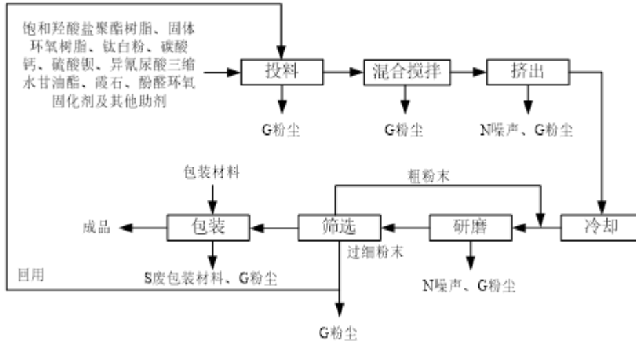
图 4.2 普鲁胺胺工艺流程
